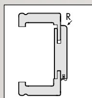
PZ-2 R Ausführung profilierte Beklei- dungen, runde Futterplatte
